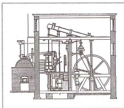
Чертёж двигателя паровой машины Дж. Уатта. XVIII в.
